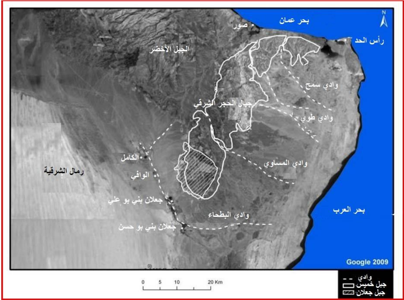
شكل (٣) جيولوجية منطقة الدراسة
